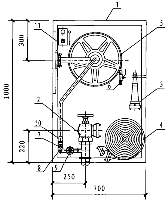
I-I 剖面图
