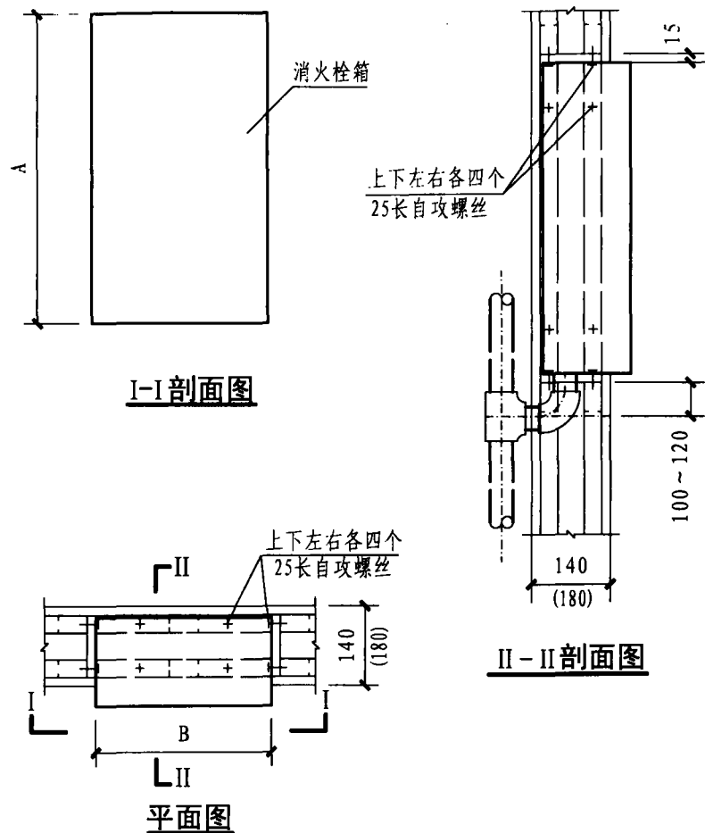
半暗装消防栓箱轻钢龙骨石膏板墙上安装固定图
