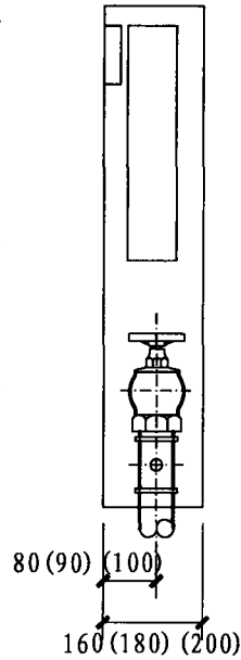
II-II 剖面图
