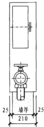
II-II 剖面图
