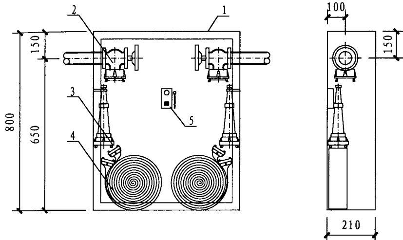
II-II剖面图
