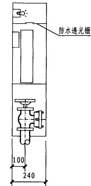
II-II 剖面图
