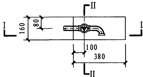
平面图
