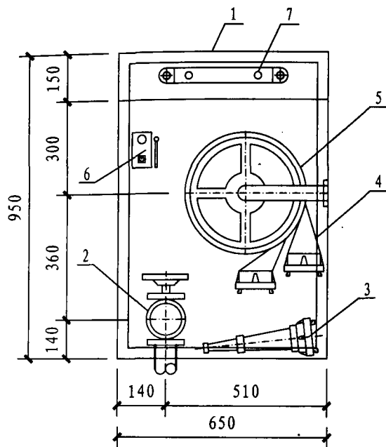
I-I 剖面图
