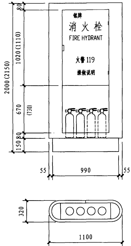
组合式消防柜外形图
