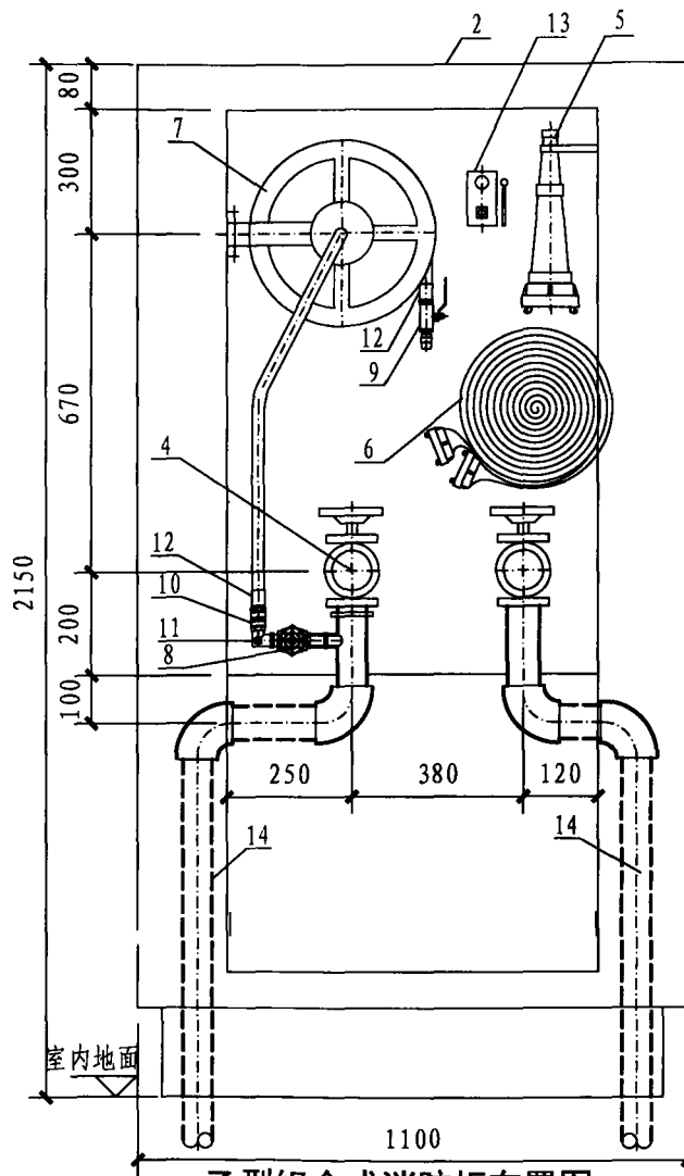
乙型组合式消防柜布置图
