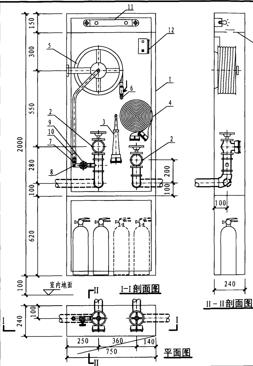
丁型带应急照明及灭火器箱组合式消防柜
