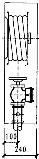
II-II 剖面图
