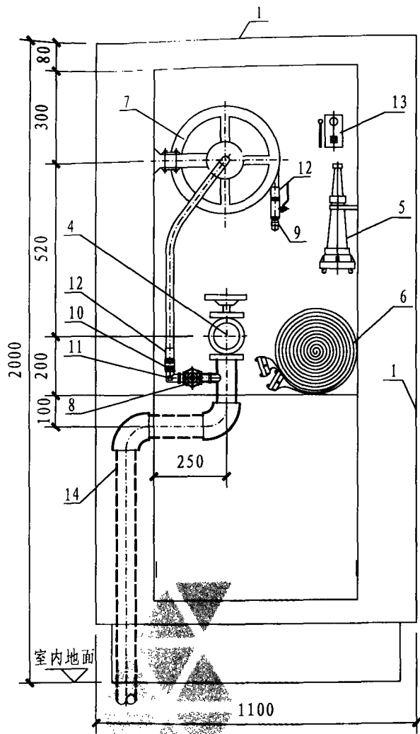
甲型组合式消防柜布置图
