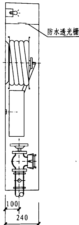
II-II 剖面图
