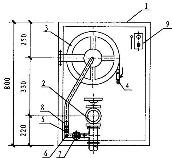
I-I 剖面图
