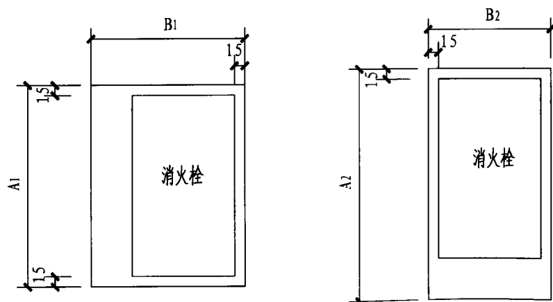
侧面进水栓箱暗装留洞图
